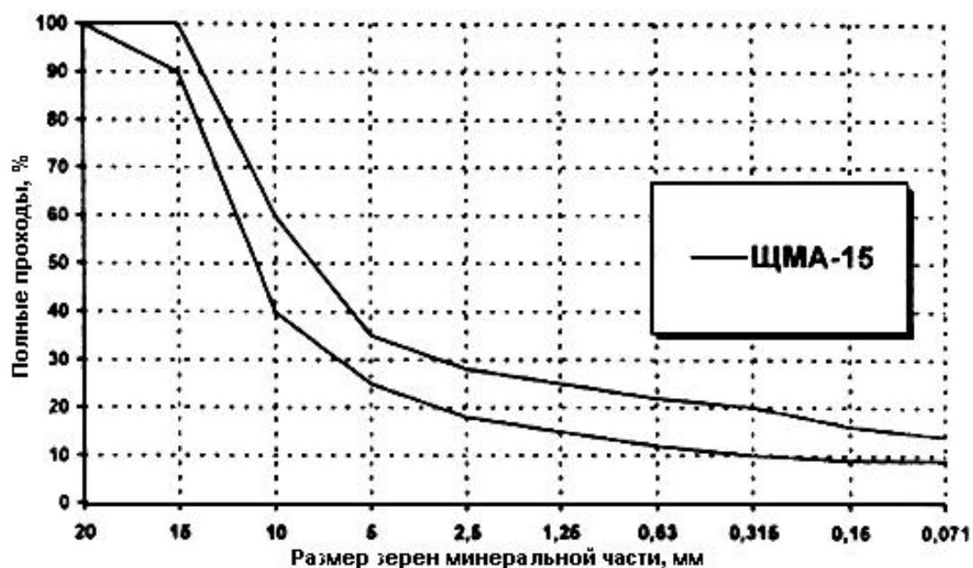
Рисунок Б.2 - Зерновой состав минеральной части ЩМА-15
